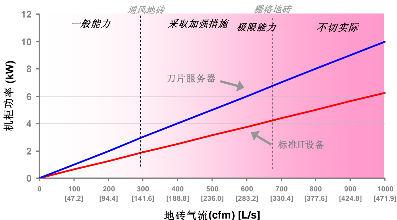
图3 - 地板砖通风气流能够为机柜提供的可用散热能力
